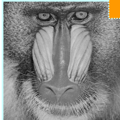
PSNR: 50.98 dB
